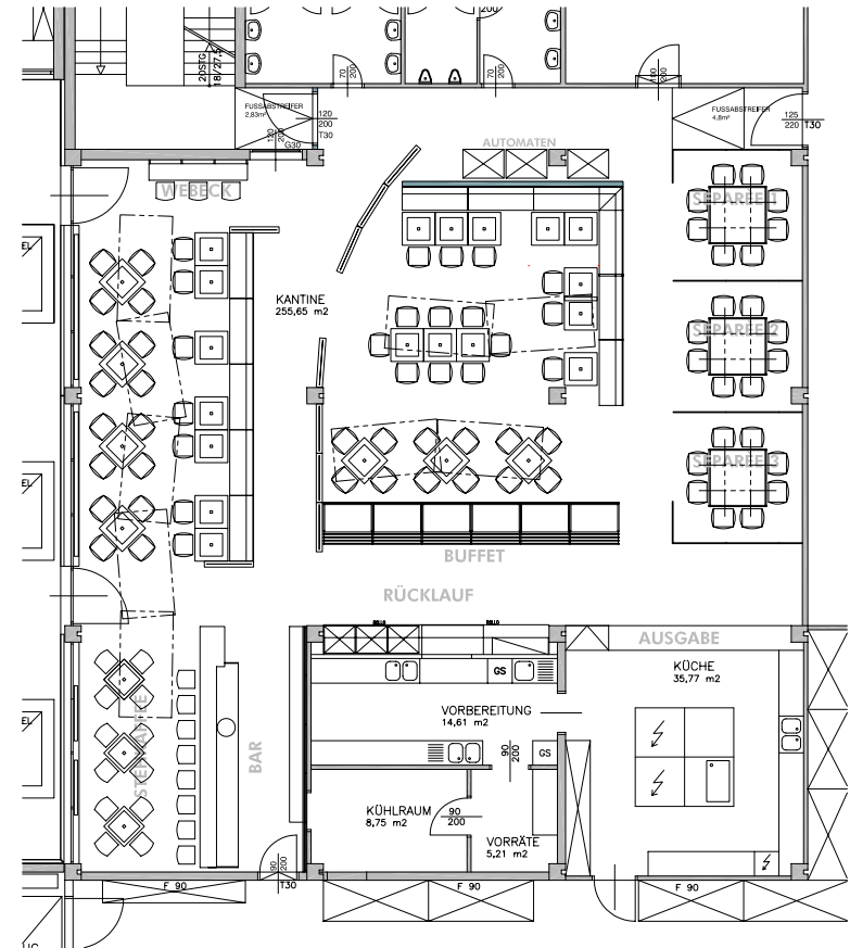
grundriss (mit lichtsegeln)
