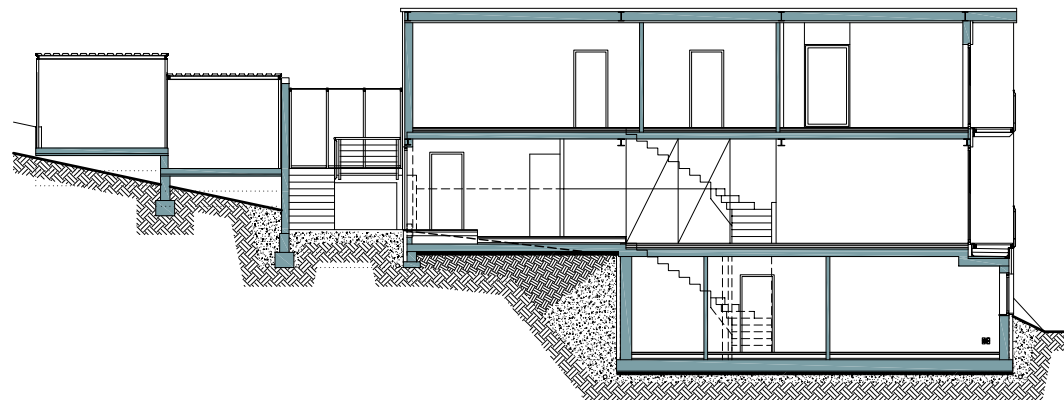
längsschnitt
