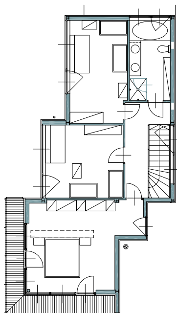
grundriss og
