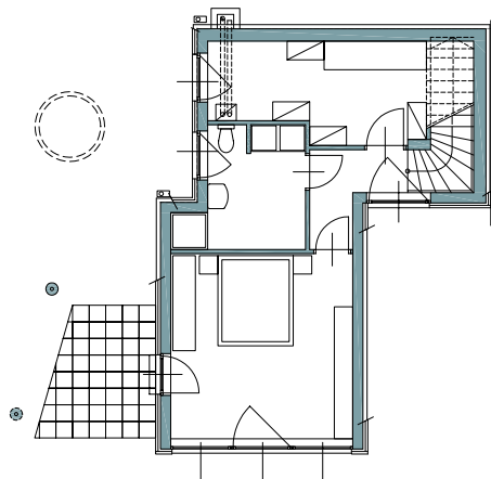
grundriss ug
