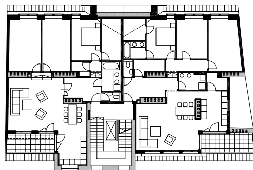
grundriss dg1
