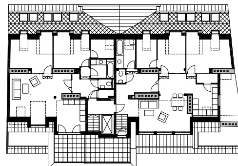
grundriss dg2
