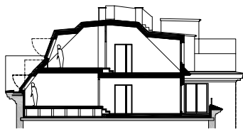
schnitt gaupen
