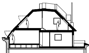
schnitt dachfenster
