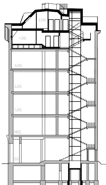
schnitt stiegenhaus
